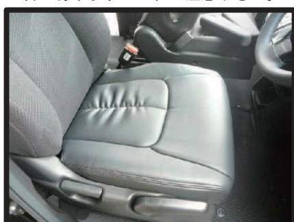
⑫カバーのラインを整え、1列目座面の完成です。助手席側も同様に取り付けます。
