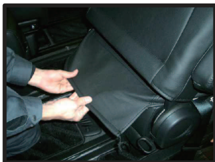
⑤入れ込んだ生地を背面から引き出します。
