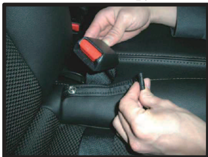
①シートベルト留め具の固定を外しておきます。
