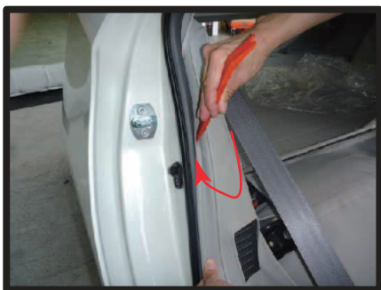
③矢印のようにサイドパーツを生地で 巻き込みます。車体とサイドパーツ の隙間に生地を入れ込みます。
