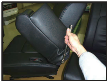
⑭アームレストを本体に戻します。 外した時と逆の手順で固定します。
