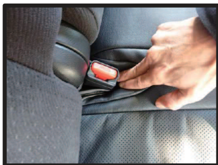
⑪シートベルトバックルの付け根に生地を入れ込みます。
