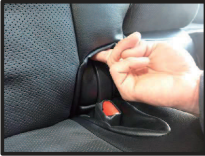
⑬図のヒンジ部分に生地を入れ込みます。
